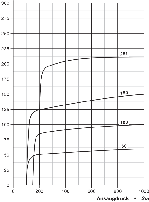
Auswahldiagramm • Selection diagram 50 Hz
